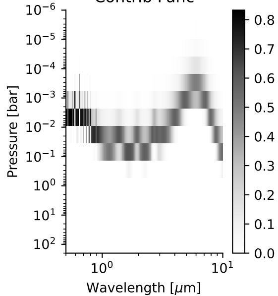
Contrib Func
